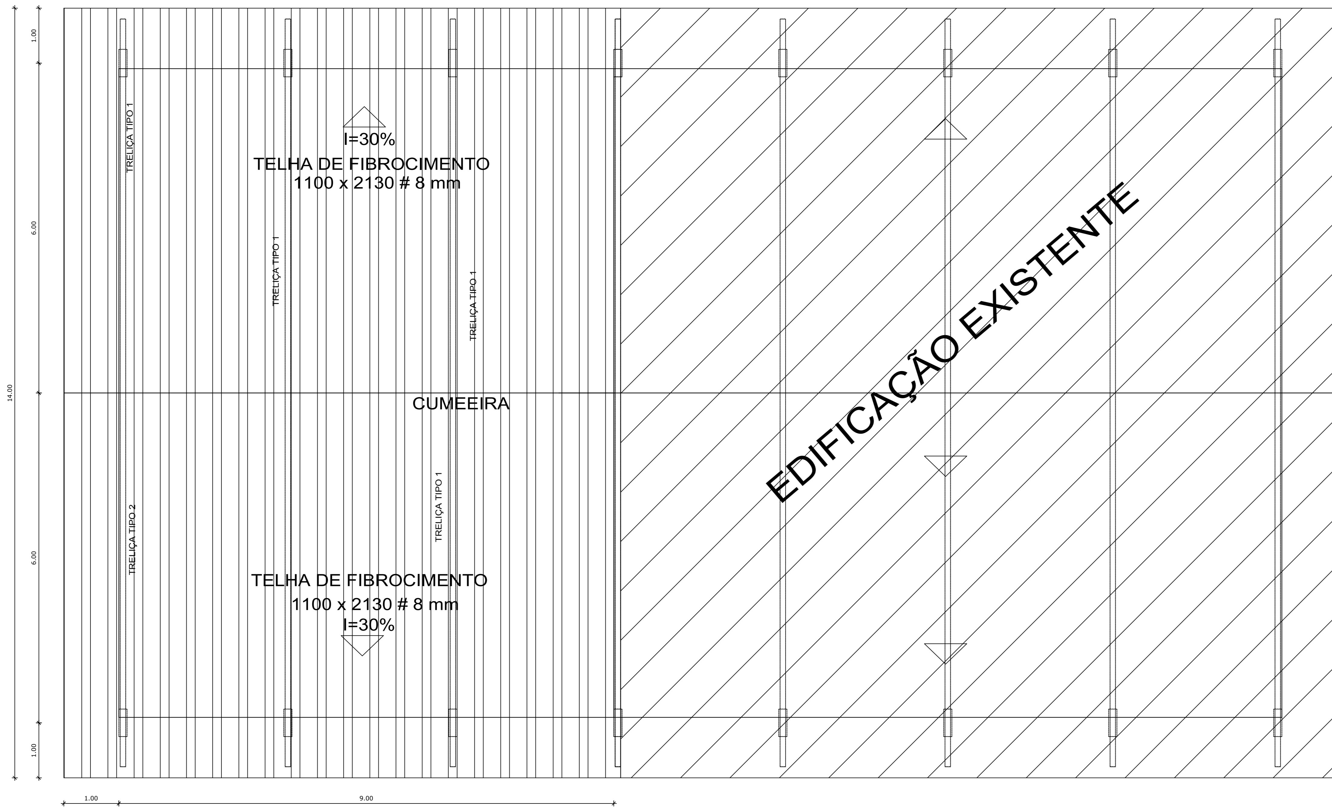
PLANTA COBERTURA ESC. 1:50
